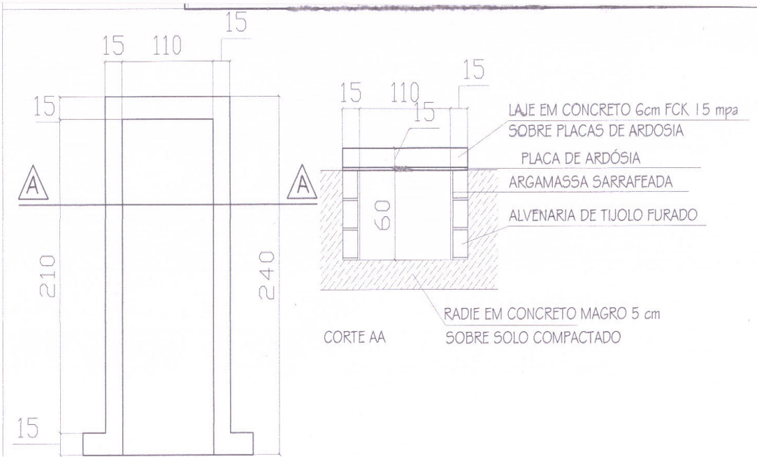
PLANTA BAIXA
